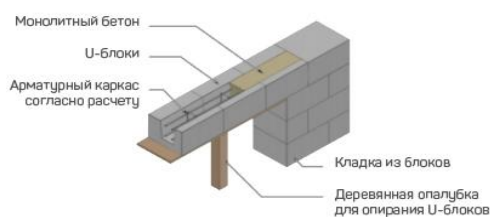
Схема изготовления перемычки из U-блоков «ЭКО»
