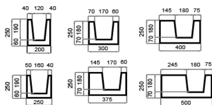
Схема изготовления U-блоков «ЭКО»
